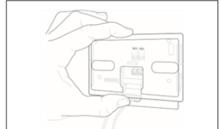
Afb. 3 De REMOCON NET MINI voorlopig op de plaat bevestigen met behulp van de daartoe voorziene haken.
