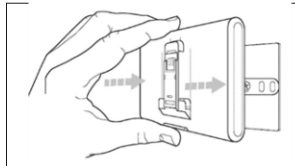
Abb. 5 Nehmen Sie das REMOCON NET MINI aus der provisorischen Position (Abb. 2) und befestigen Sie das Gateway an der Platte, indem Sie auf die Seiten drücken, bis das Einrasten der vier gleichen Seitenhaken nicht mehr zu spüren ist.
