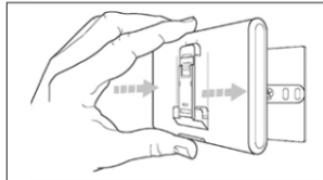
Afb. 5 De voorlopig aangebrachte REMOCON NET MINI (afb. 2) verwijderen en het apparaat op de plaat bevestigen door stevig op de zijkanen te drukken totdat u de vier kleine haakjes aan de zijkanen hebt horen klikken.
