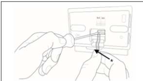
Abb. 4 Verbinden Sie das Adempaar des Steckers BUS BridgeNET auf der Heizplatte mit dem Anschluss BUS BridgeNet des REMOCON NET MINI (unter Beachtung der Polarität B mit B und T mit T)*.
