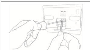
Fig. 4 Forbind ledningssparret fra konnektoren på BUS BridgeNet-kortet på fyret til BUS BridgeNet på REMOCON NET MINI-konnektoren (overhold polariteten B med B og T med T)*. * plastikflanen kan fjernes for at lette tilslutningen af ledningerne, sådan som vist i figuren.
