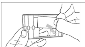
Fig. 1b Sæt den dobbeltklæbende tape bag holdepladen, fjern den beskyttende film og gør den fast på fyrets metalplade.
