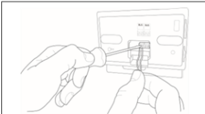
Afb. 4 Het dradenpaar van de BridgeNet BUS-connector op de ketel-kaart met de BridgeNet BUS-connector van de REMOCON NET MINI verbinden (de polariteit B met B en T met T in acht nemen)*
